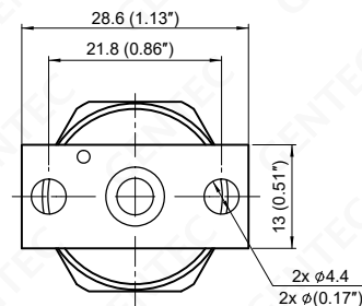
C-Seal 单孔
